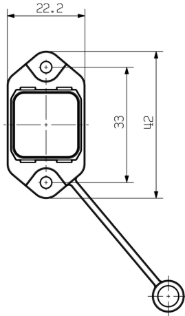
Rysunek wymiarowy
