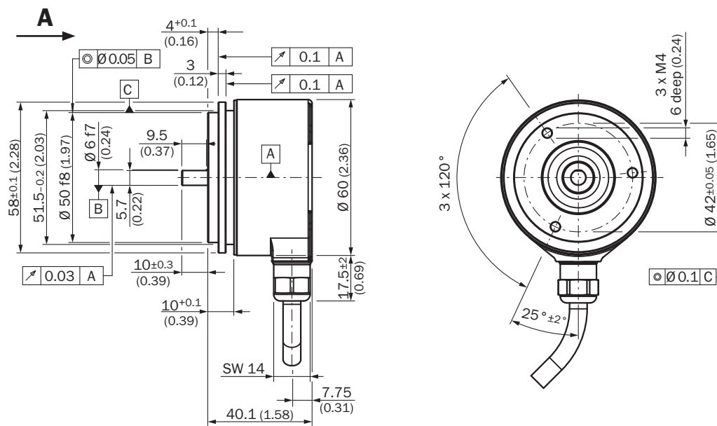
Rysunek wymiarowy (Wymiary w mm)
