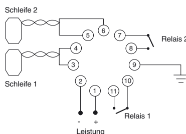
11-poliger Stecker
